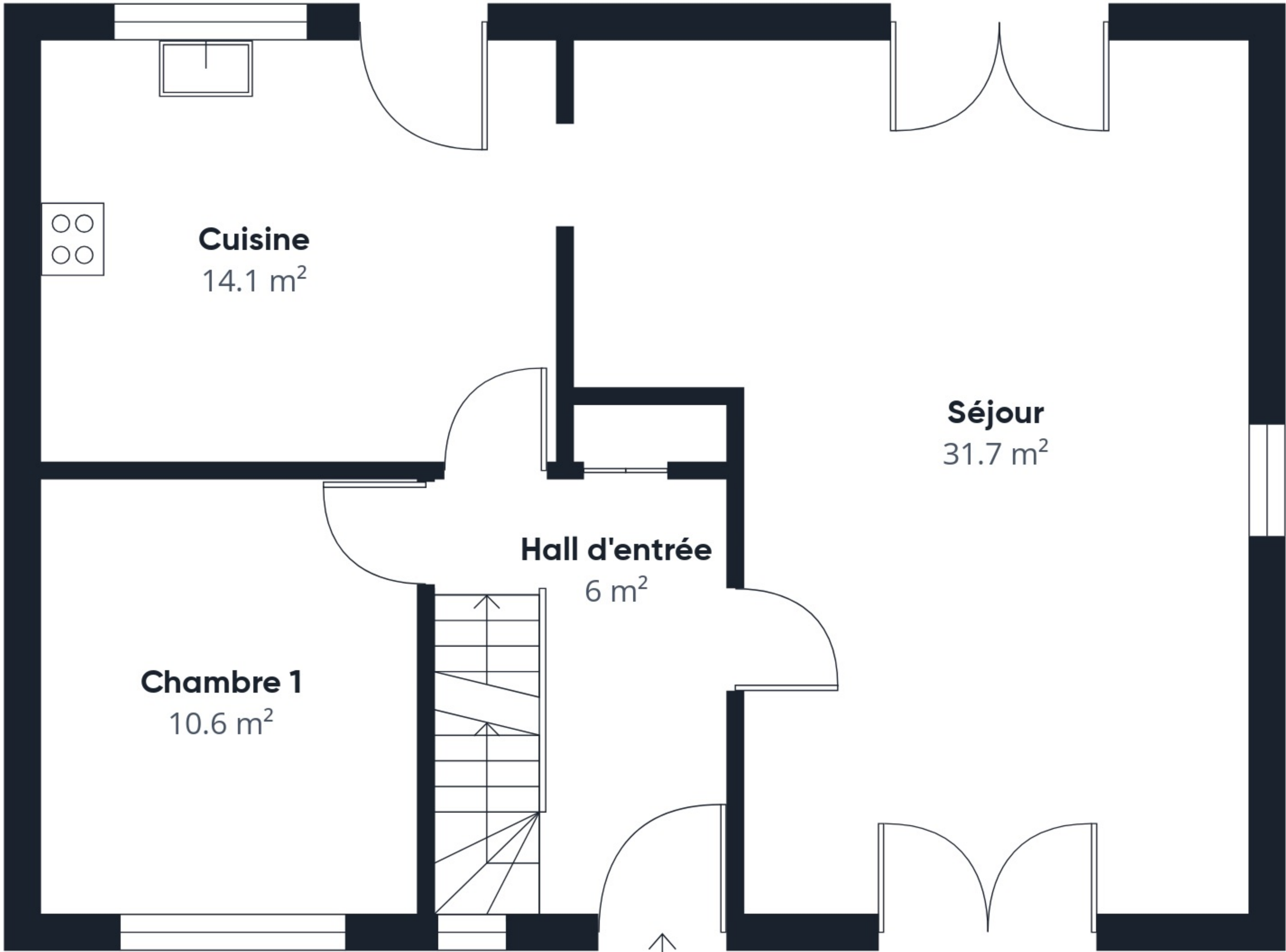
Niveau 0
